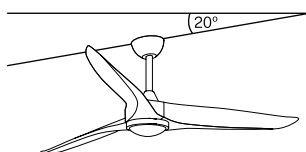
Montaggio ad angolo
