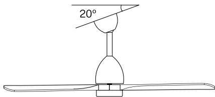
Hoek montage
