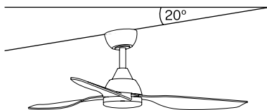
Hoek montage
