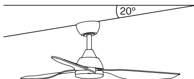
Winkelmontage
