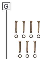
SCHRAUBEN + UNTERLEGSCHLEIBEN FÜR DIE KLINGEN
